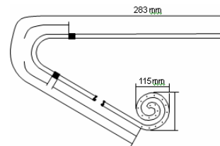
Tenckhoff Pediátrico Swan Neck em espiral 283/115
